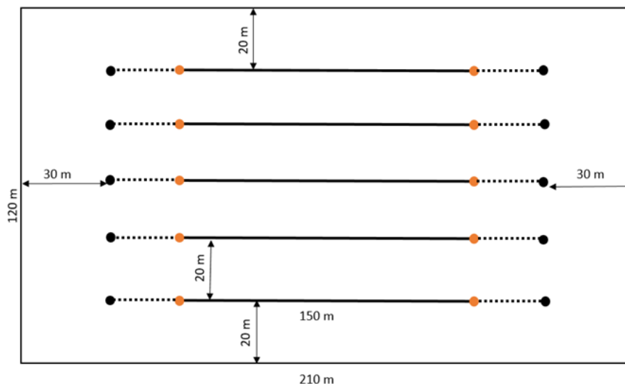
Figuur 4-2 : Inplanting van één plot.
