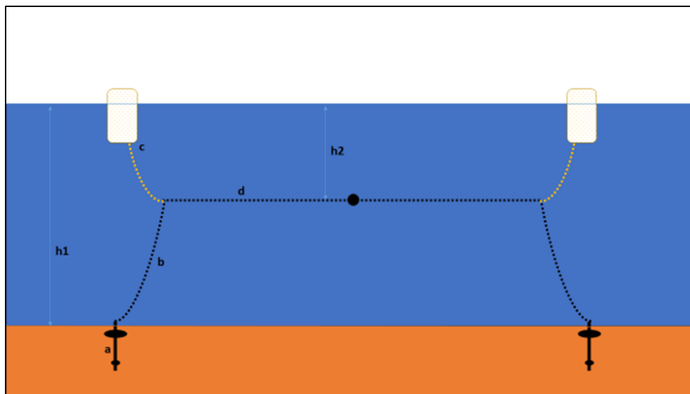
Figuur 4-1: Schematische voorstelling van de hoofdlijn met verankering voor de kweek van schelpdieren en zeevieren bij doodtij en hoogwaterstand. a) schroefanker, b) ankertouw, c) hoekboei, d) hoofdlijn of backbone h1) de zone Westdiep is gemiddeld 12m diep, h2) de hoofdlijn wordt op 1-2 m onder het zeewateroppervlak gehouden.
