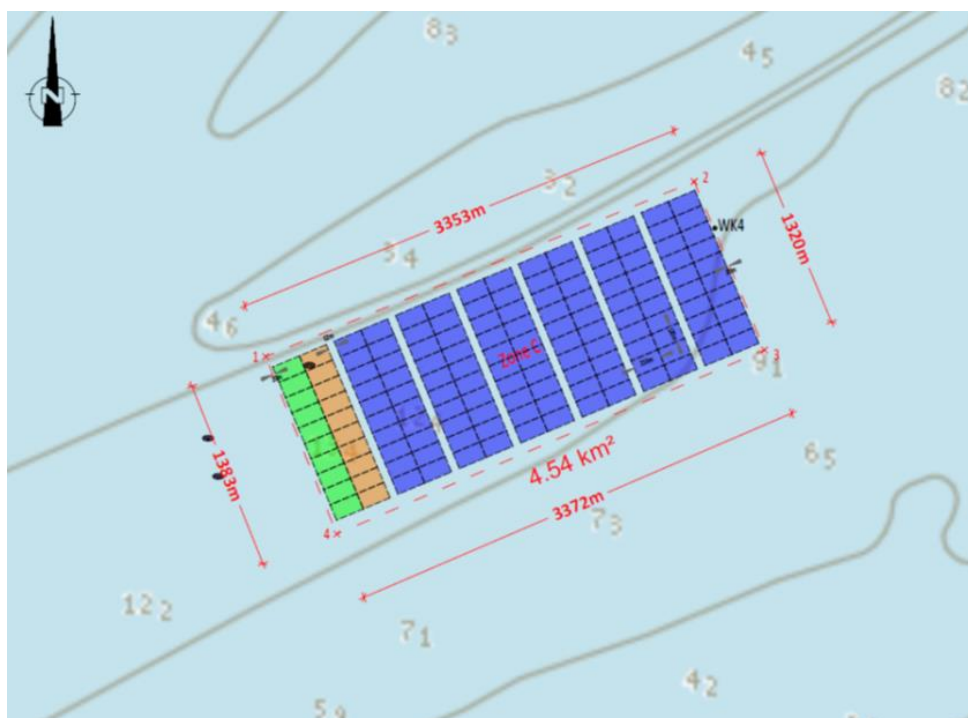
Figuur 4-3 : Indeling van de volledige productiezone. Groen: productie zeewier, Oranje: productie oesters, Blauw: productie mosselen.
